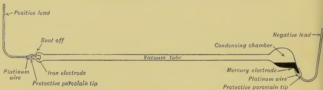
FIG. 200.—Cooper-Hewitt Mercury Vapour-lamp.
